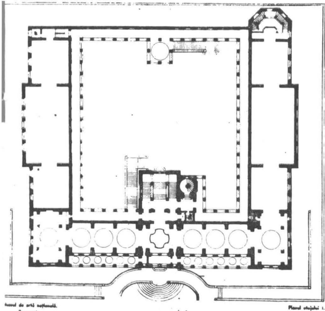
Planul etajului I.
