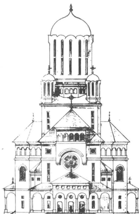
PROIECTUL UNEI CATE- DRALE LA BUCUREȘTI (1936): 4. Plan — 5. Fațada principală — 6. Secțiune — 7. Machetă
