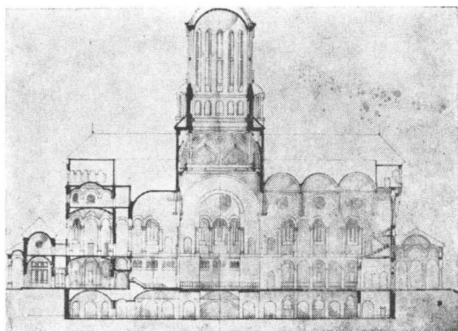
PROIECTUL UNEI CATE- DRALE LA BUCUREȘTI (1936): 4. Plan — 5. Fațada principală — 6. Secțiune — 7. Machetă
