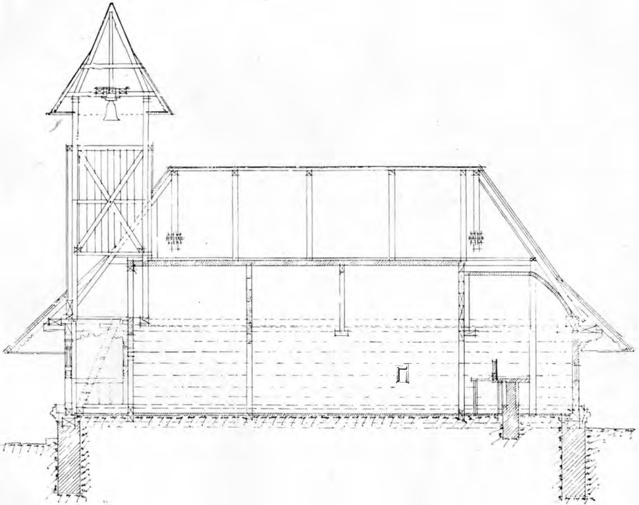
Biserica Sf. Nicolae Dobrușa-de-jos, Vâlcea. Secție longitudinală.
