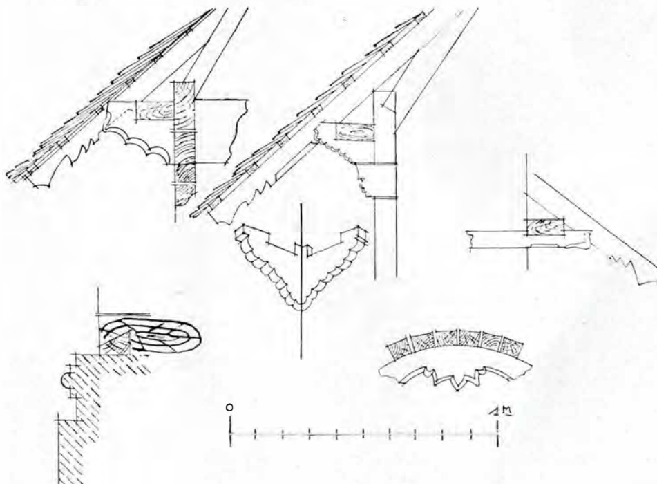
Biserica Sfântul Nicolae Dobrușa-de-jos, Vâlcea. Detalii.
