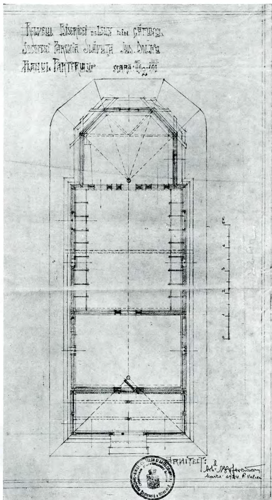
Biserica Slăvuța-Socoleni, Dolj. Planul.
