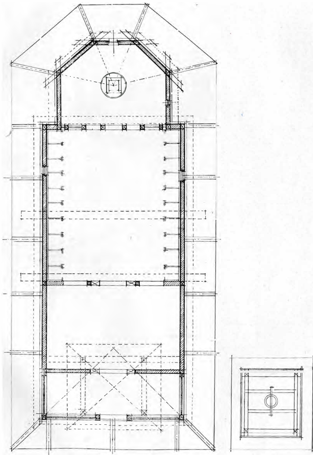
Biserica Sf. Nicolae, Dobrușa-de-jos, Vâlcea. Planul.
