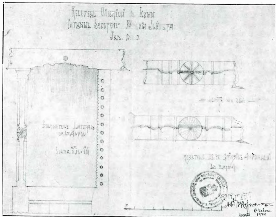
Biserica Slăvuța-Socoteni, Dolj. Detalii.
