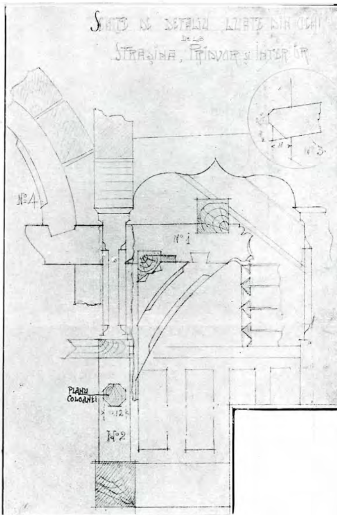
Biserica din Grămești-Pielreni, Vâlcea. Detalii din strașină.
