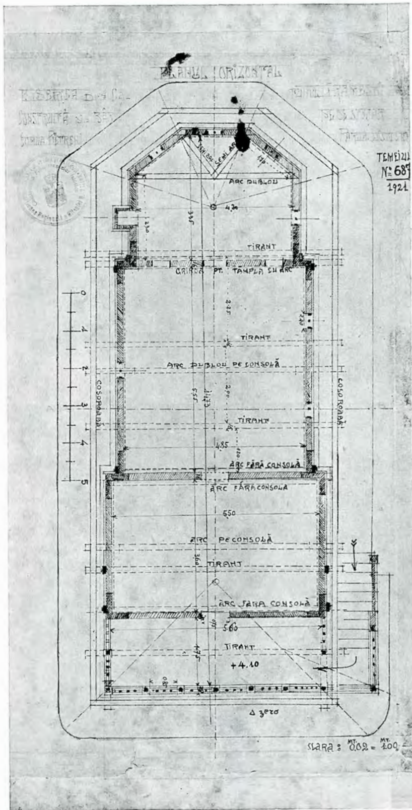
Biserica din Grămești-Pietreni, Vâlcea. Planul.
