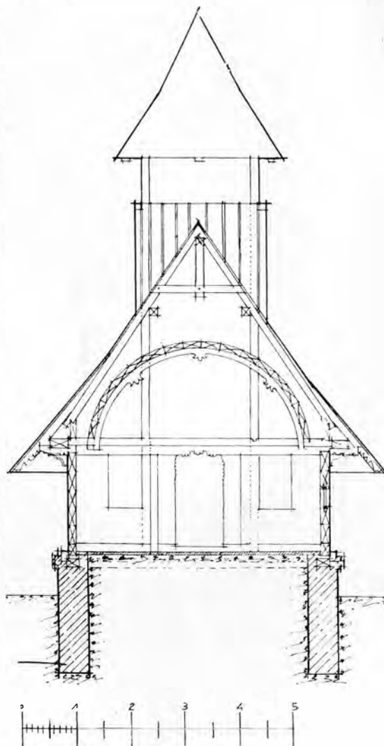
Biserica Sfântul Nicolae, Dobrușa-de-jos, Vâlcea. Secție transversală.
