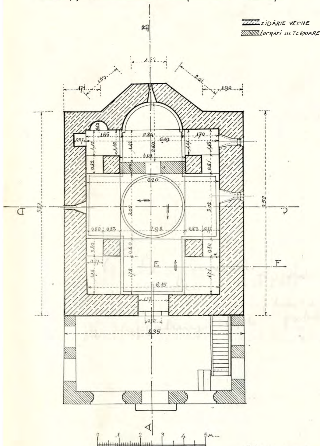
Fig. 3. — Planul orizontal.
