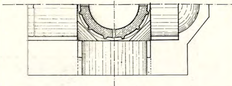
Fig. 10. — Planul bolților și al turlei.
