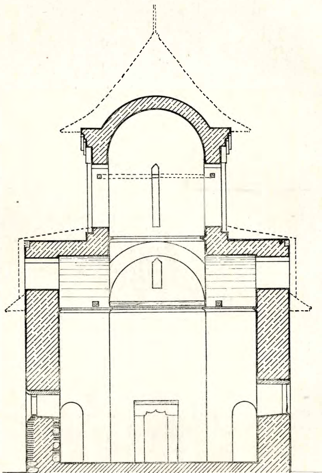
Fig. 9. — Secția transversală C. D.
