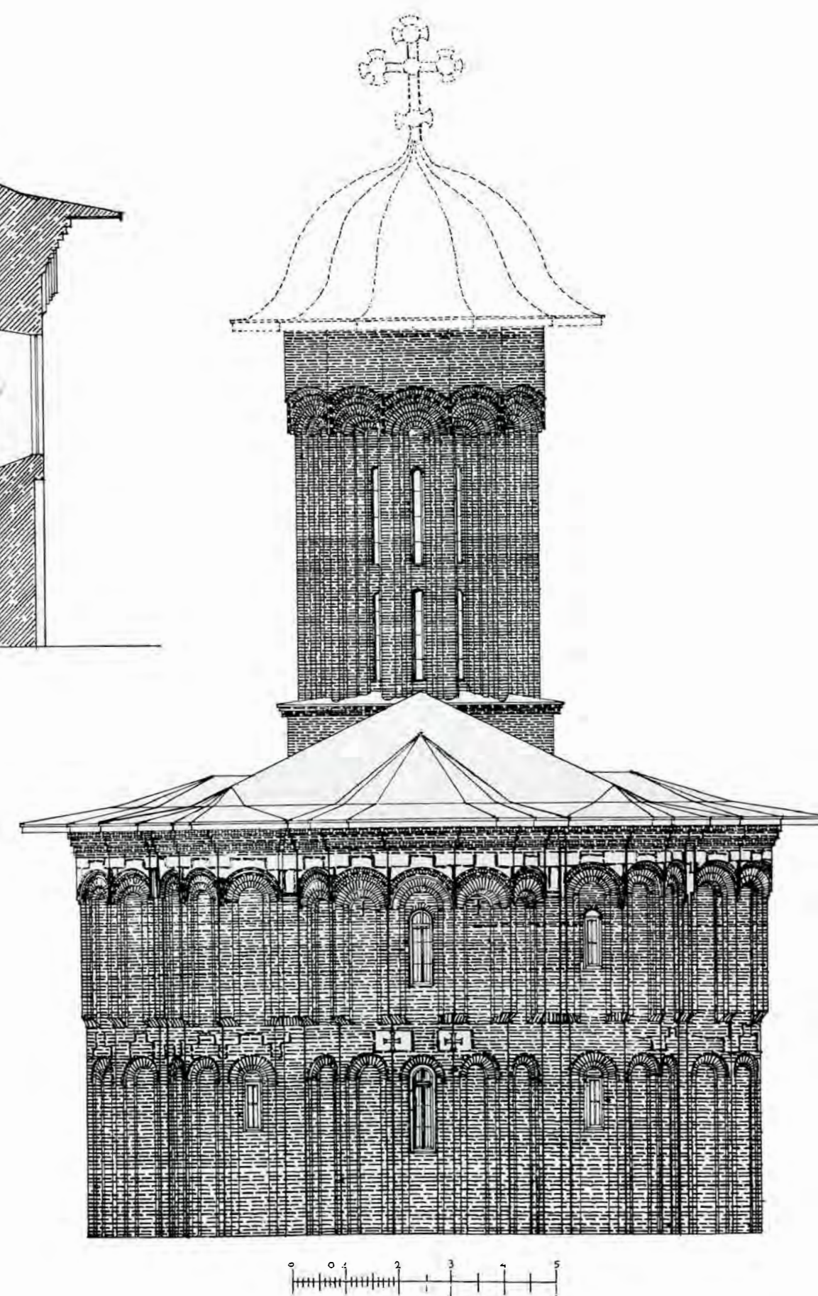
Fig. 102.— Fațada spre altar a bisericii de la fosta
