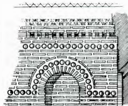
Fig. 86.— Detalii de fațadă la absidă.
