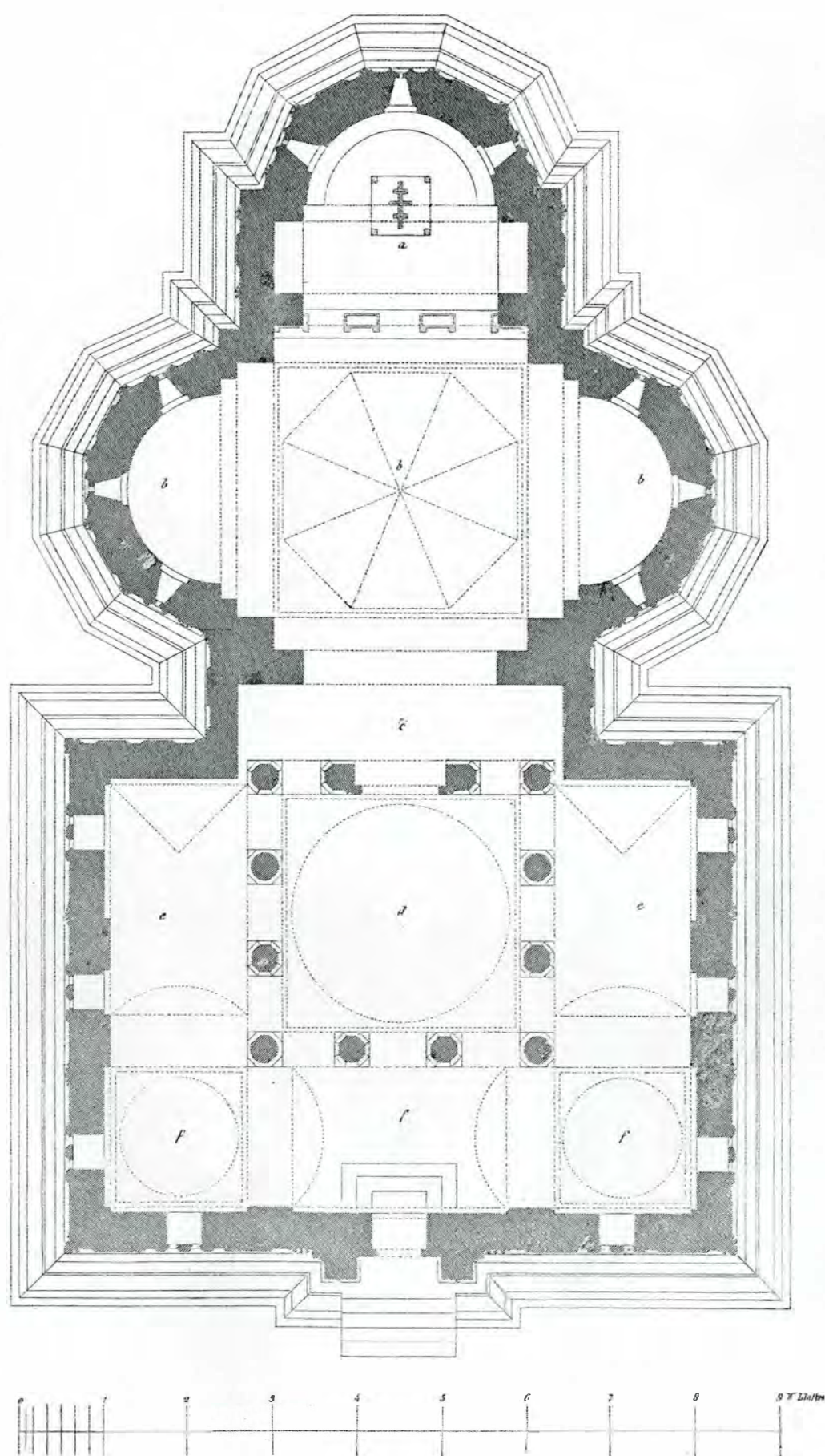
Fig. 143.— Biserica Episcopală de la Curtea de Argeș. Planul original al Măsterului Manole.
